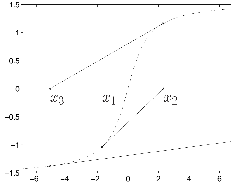
Divergenz des Newtonverfahrens, f(x) = \arctan x
